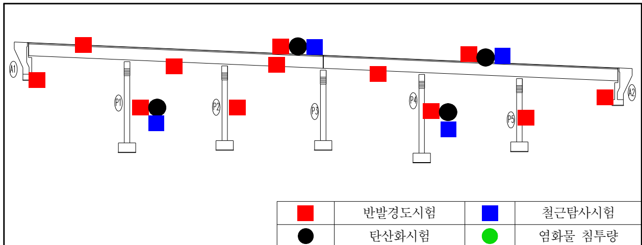
【그림 3.4.2】 콘크리트 내구성조사 위치도(영천방향)
