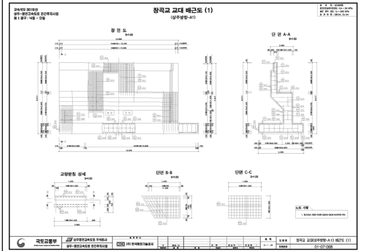
【그림 3.1.13】 교대 배근도
