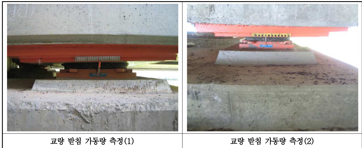
【사진 3.3.40】 교량받침 이동량 측정
