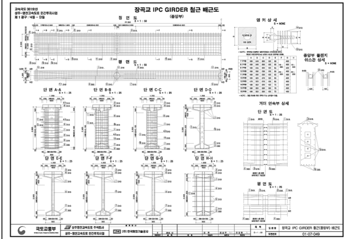
【그림 3.1.12】 거더 배근도
