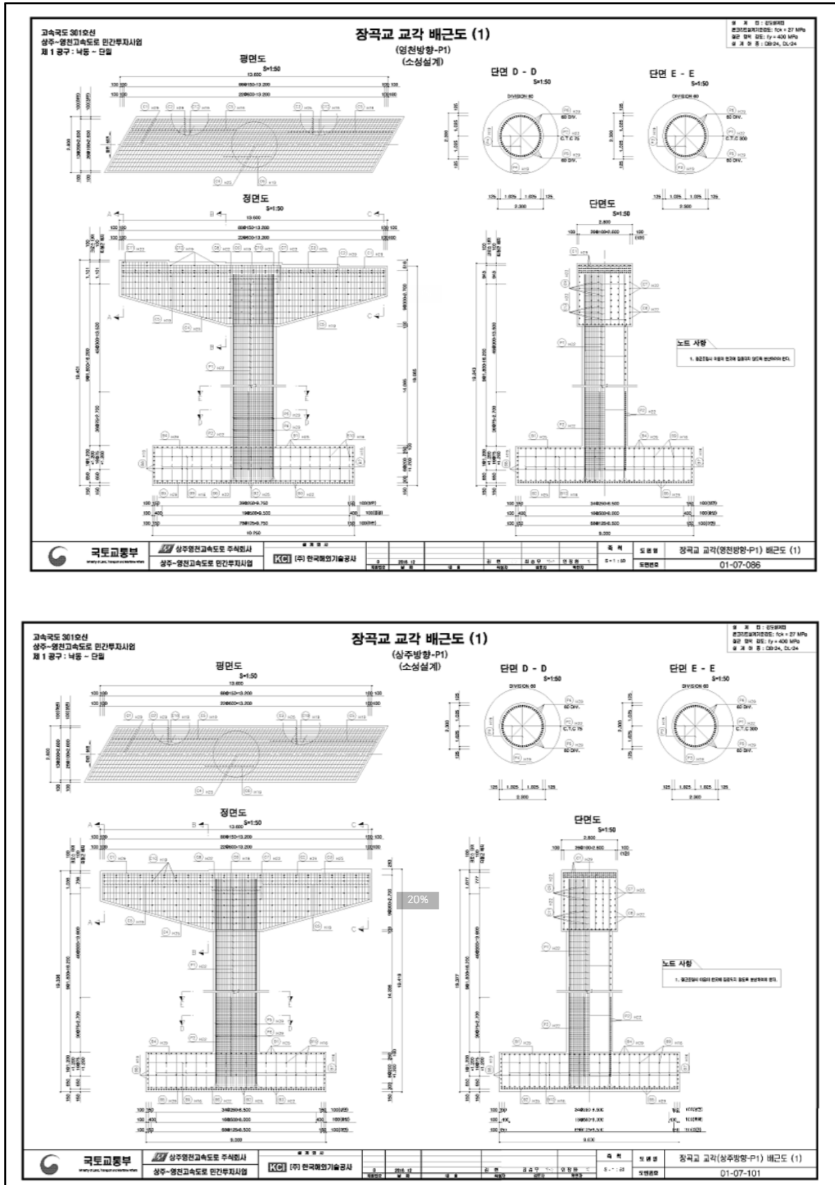
【그림 3.1.14】 교각 배근도
